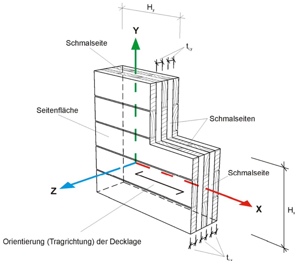
Abbildung 6: Haupttrichtungen infolge Belastung in der Ebene der Massivholzplatte
