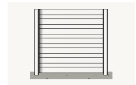
Abbildung 5: waagrechte lückenlose Belattung, Ansicht
