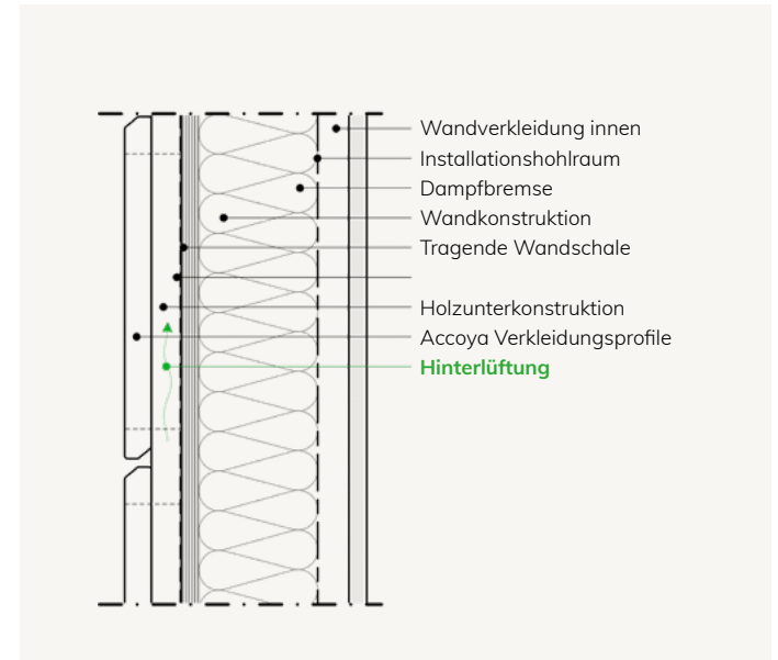
Abbildung 1: hinterlüftete Fassadenverkleidung, Systemskizze
