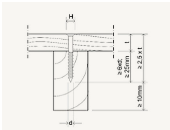
Abbildung 5: Die empfohlene Eindringtiefe der Schrauben in die Unterkonstruktion beträgt mindestens 25 mm oder das Sechsfache des Schaftdurchmessers der Schraube oder das 1,5-Fache der Dielendicke (je nach dem, welcher Wert der größte ist).
