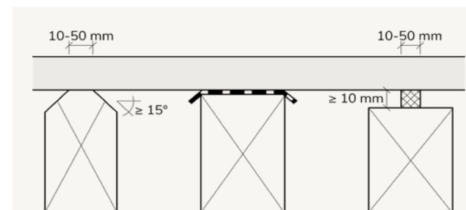
Abbildung 3: Unterkonstruktion (Detailansicht)
