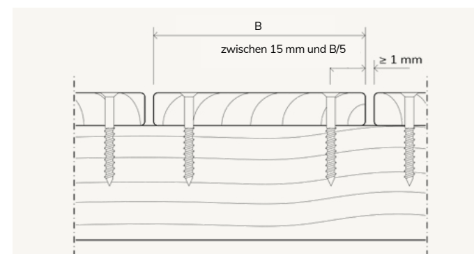
Abbildung 4: Der Abstand zu den Längsseiten der Dielen liegt zwischen 15 mm und 1/5 der Dielenbreite
