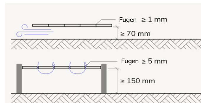
Abbildung 2: Anforderungen an die Belüftung
