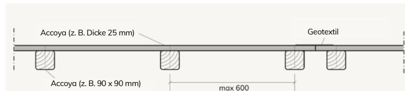
Abbildung 2: Querschnitt
