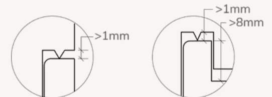
Abbildung 3: Abstandswulst (Detailansicht)
