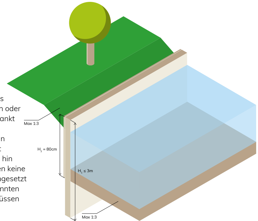
Abbildung 1: Längsschnitt
